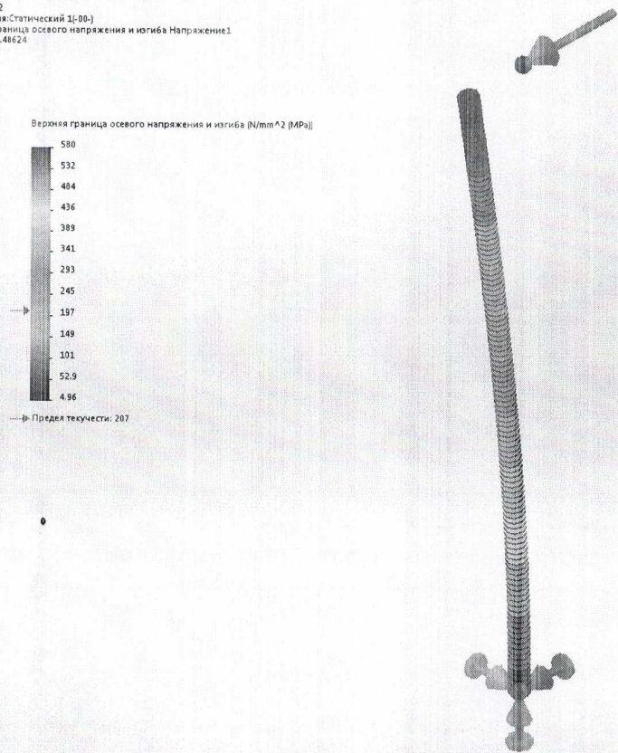
Труба 76x2-Статический 1-Напряжение-Напряжение1
