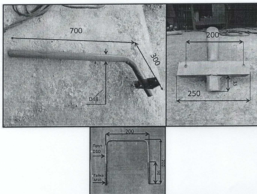
Рис.1 – Эскиз кронштейна
