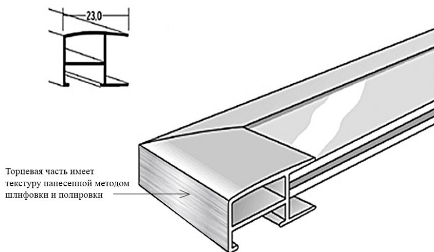
Рисунок 2. Алюминиевый профиль Nielsen №62 202004
