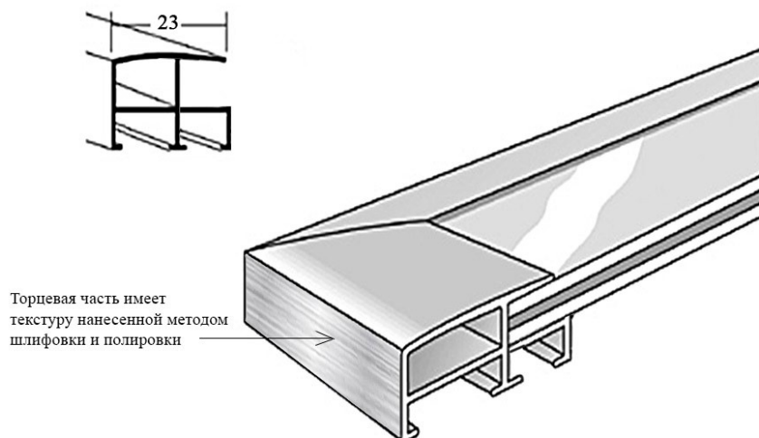
Рисунок 4. Алюминиевый профиль «KRAUSS №02 202004»
