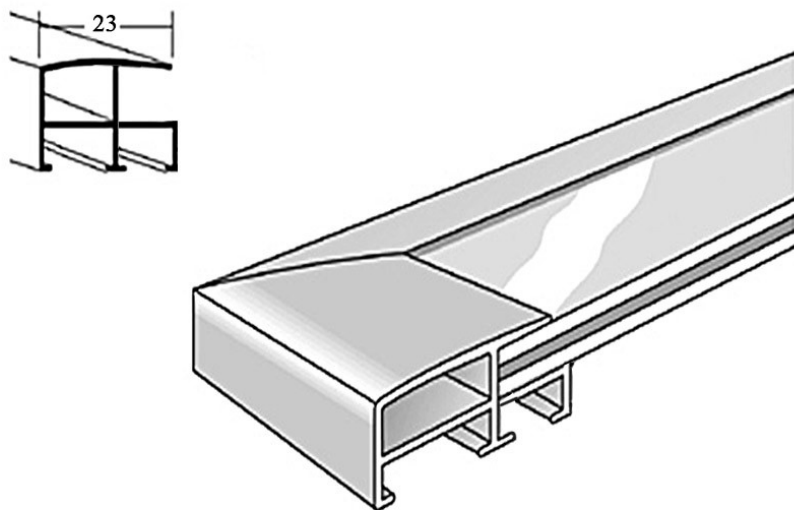
Рисунок 3. Алюминиевый профиль пн-62 анод.мат. серебро 3.05»
