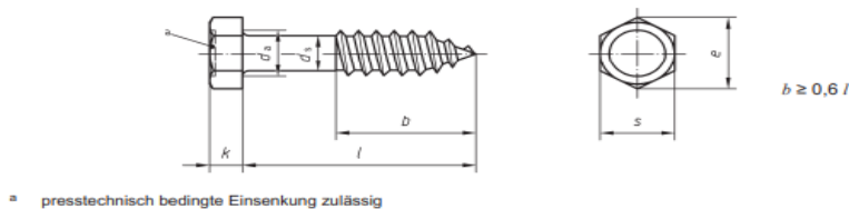
Bild 1 — Sechskant-Holzschraube
