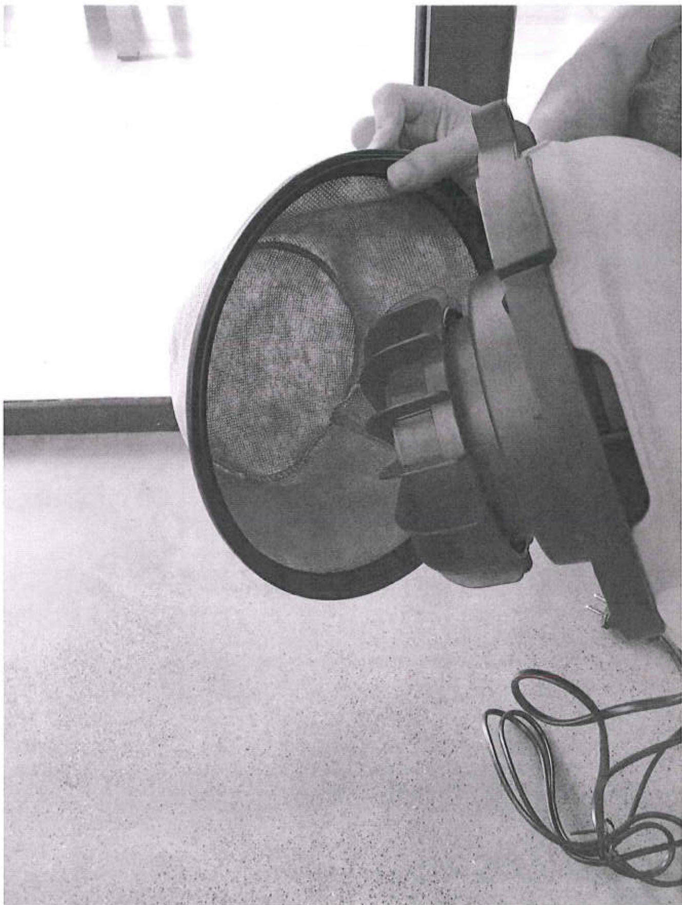
Двухступенчатая фильтрация в сборе на моторном отсеке.
