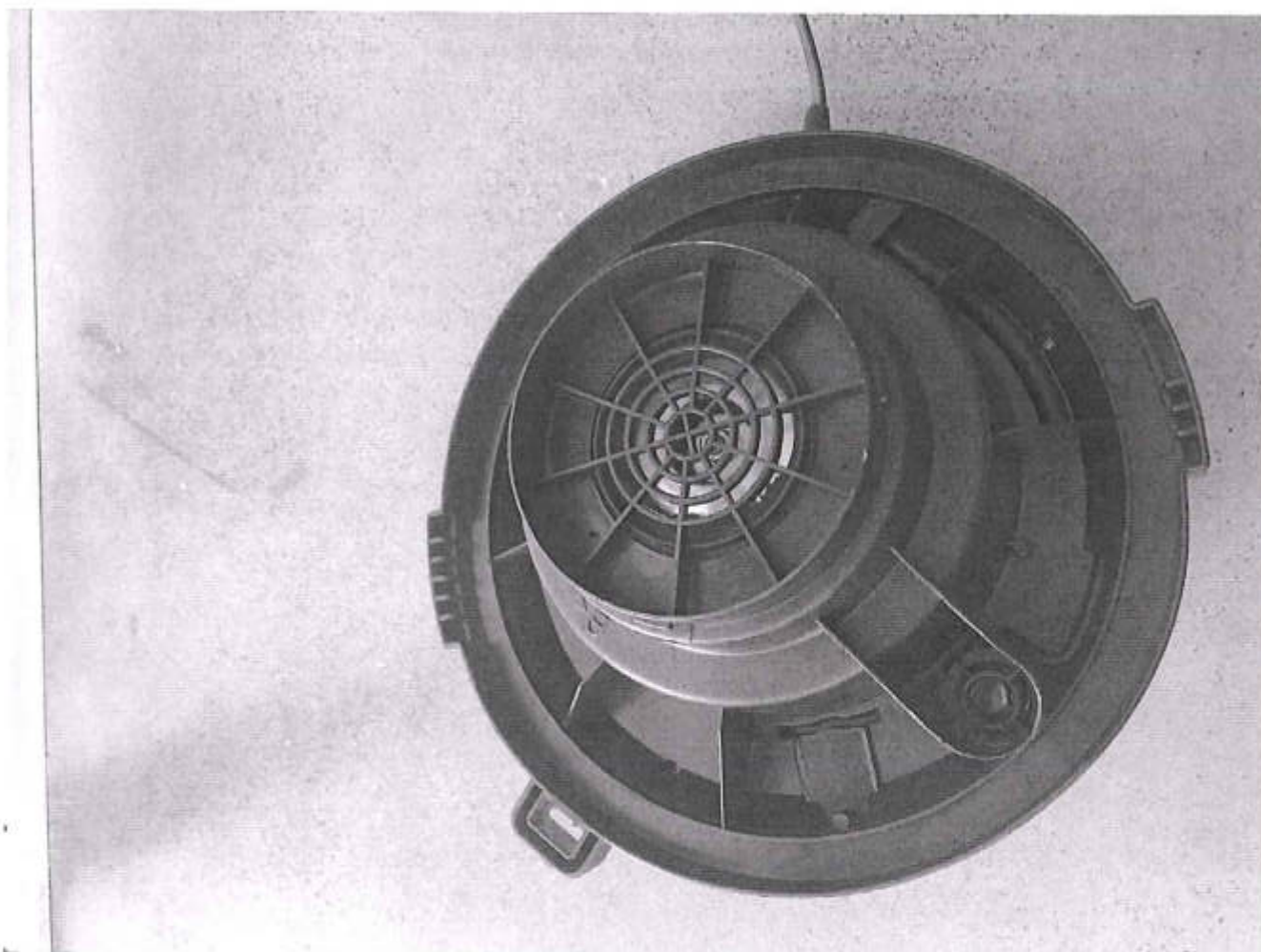
Моторный отсек.
