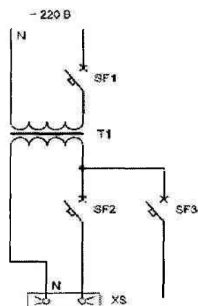
Рис. 13.2.1. Схема принципиальная ящика серии ЯТП.
